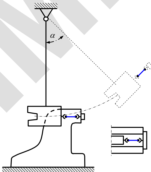
Rys. 6. Schemat próby udarowego rozciągania przy użyciu młota wahadłowego
