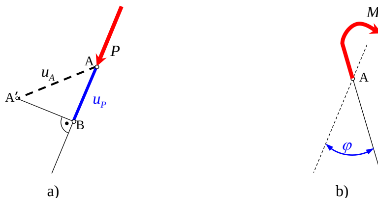
Rys. 1. Przesunięcie odpowiadające: a) sile skupionej P ; b) momentowi M
