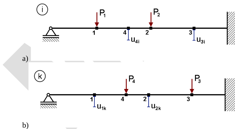
Rys. 7. Doświadczalna weryfikacja twierdzenia Bettiego
