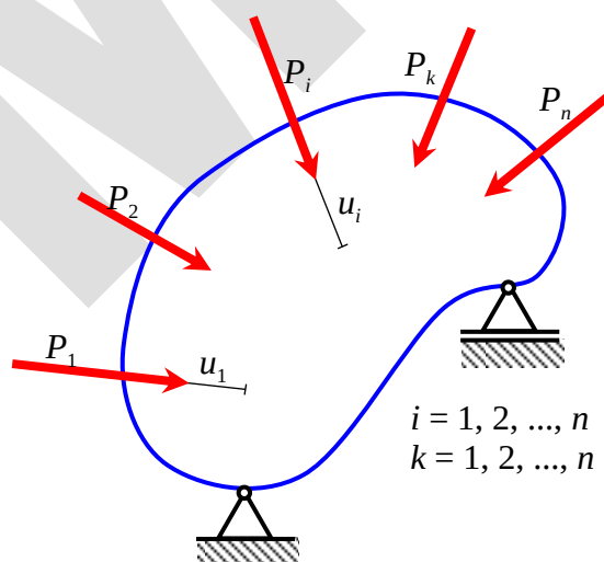
Rys. 2. Ciało liniowosprężyste i przemieszczenia odpowiadające danym siłom skupionym
