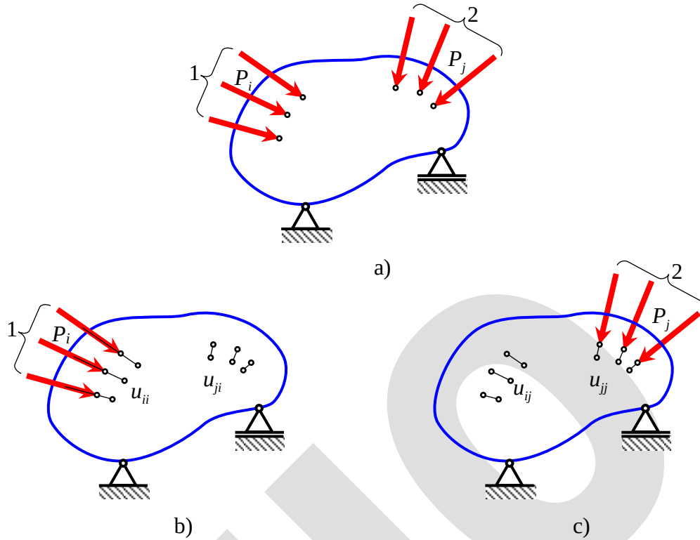
Rys. 3. Ciało liniowosprężyste obciążone dwoma układami sił
