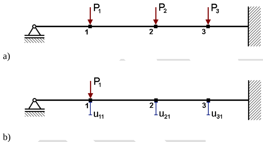
Rys. 8. Doświadczalna weryfikacja symetrii macierzy podatności
