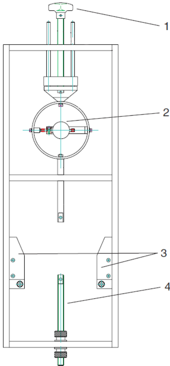
Rys. 6. Urządzenie obciążające
