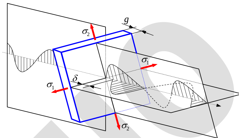
Rys. 4. Dwójłomność wymuszona
