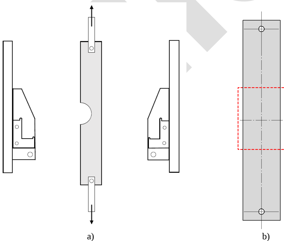
Rys. 8. Rozciąganie modeli: a) zamocowanie modelu w urządzeniu obciążającym; b) model wykorzystywany do wyznaczania elastooptycznej stałej modelowej wraz z zaznaczonym obszarem, w którym obserwowane są izochromy
