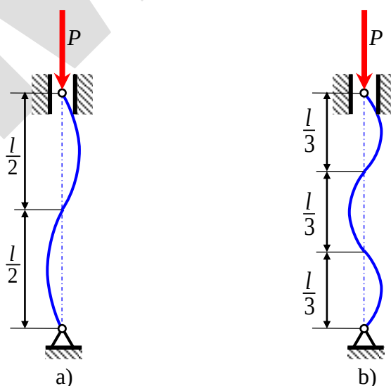
Rys. 5. Postaci wyboczenia dla a) n = 2 ; b) n = 3
