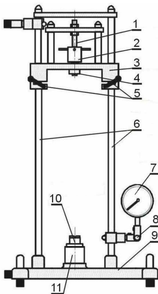
Rys. 9. Schemat stanowiska do badania prętów na wyboczenie
