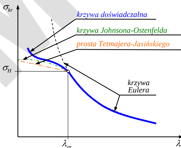
Rys. 6. Zależność naprężeń krytycznych od smukłości pręta ulegającego wyboczeniu Wartość graniczną smukłości wyznacza się z zależności:
