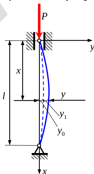
Rys. 7. Wyboczenie pręta o wstępnej krzywiźnie
