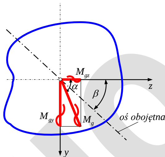
Rys. 3. Położenie osi obojętnej w zginaniu ukośnym
