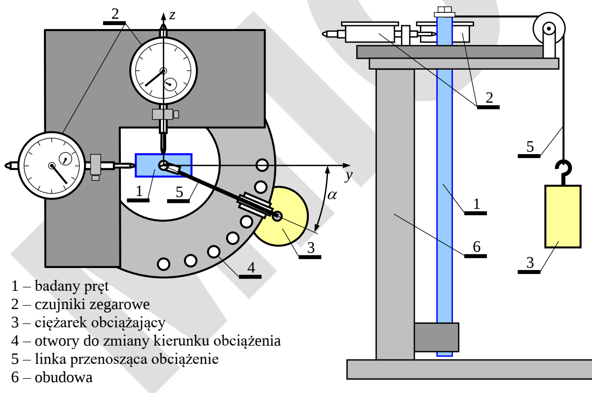
Rys. 4. Stanowisko do zginania ukośnego
