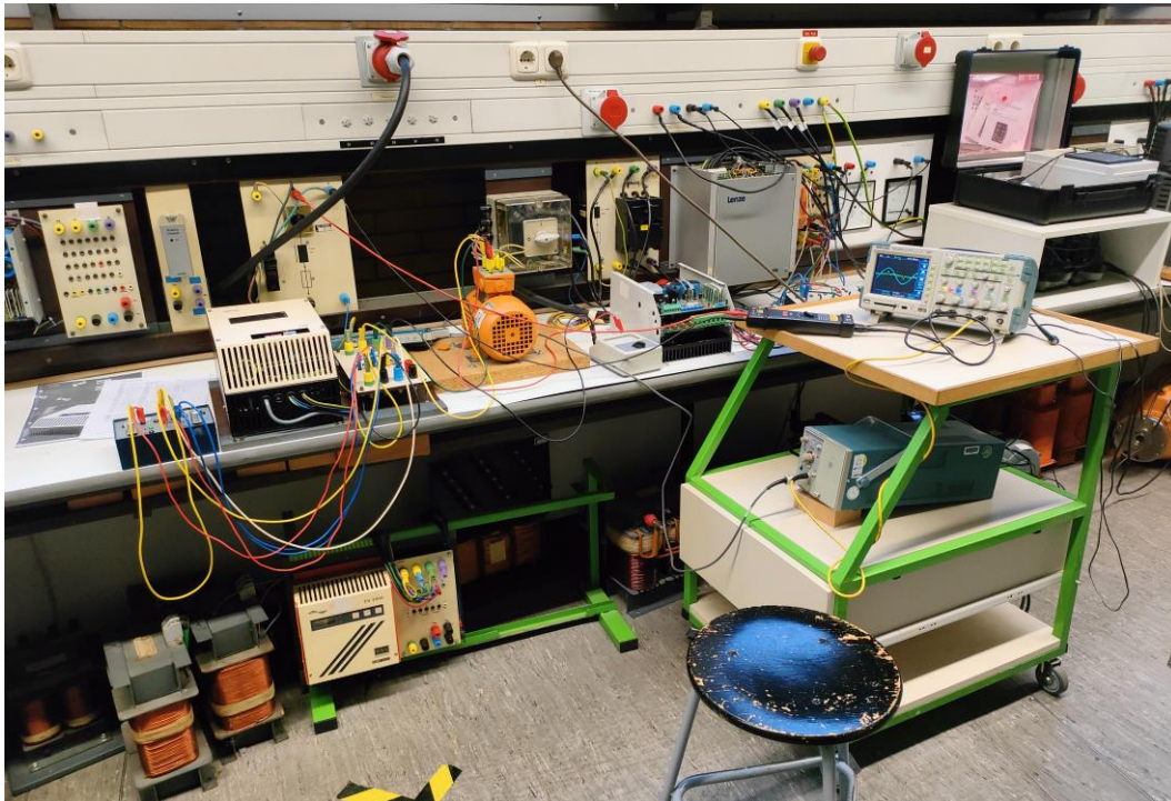
Rys. 4. Laboratorium energoelektroniki
